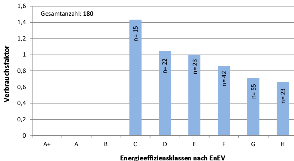
Abbildung 3.26: Verbrauchsfaktor für die untersuchten 180 Gebäude mit 7-12 Wohneinheiten und deren Verteilung auf die Effizienzklassen der EnEV (Daten aus (Fraunhofer ISI et al, 2005), eigene Darstellung)
