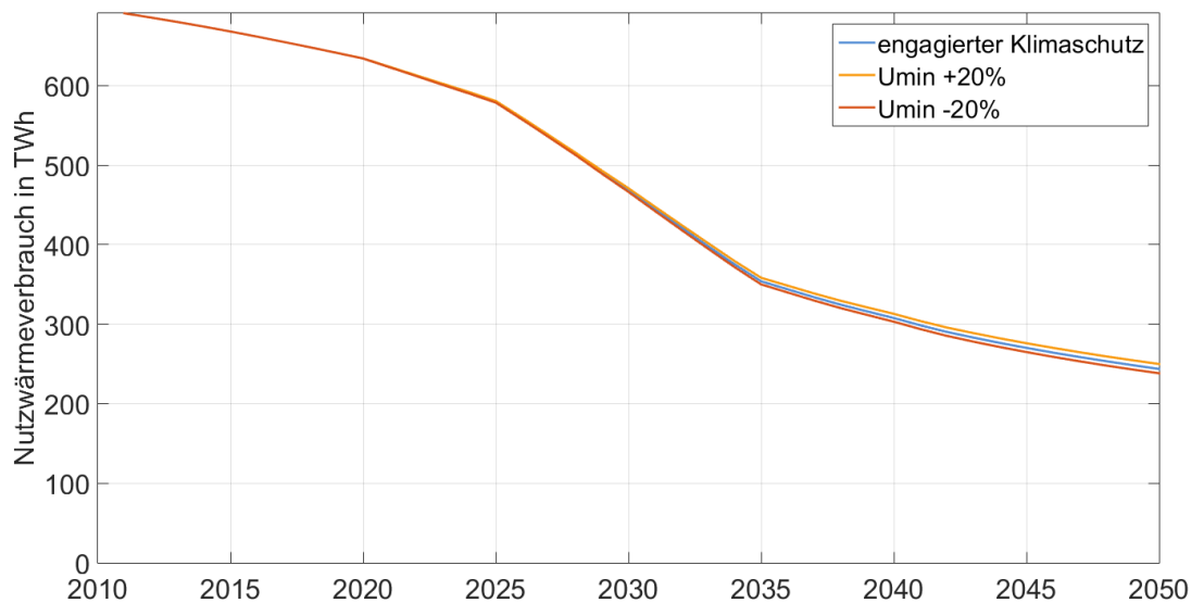
Abbildung 5.17: Sensitivität des minimal erreichbaren Wärmedurchgangskoeffizienten ( U_{\min} )
