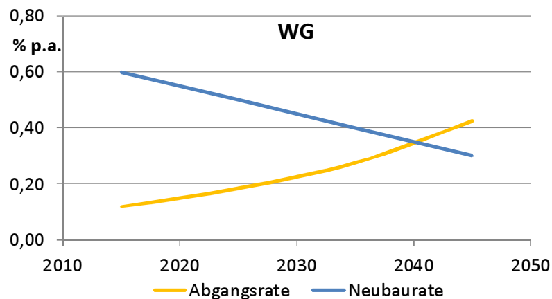
Abbildung 3.14: Variierende Abgangsraten bei vorgegebener Neubaurate. Die Abgangsrate ergibt sich aus dem jeweiligen Gesamtflächenbedarf der Bevölkerung. Im Resultat finden sich bei hoher Neubaurate in 2050 mehr energieeffiziente, neue Gebäude und weniger alte, oftmals ungedämmte Gebäude im Bestand. Bei den im Bestand verbleibenden Altbauten wird gleichzeitig von einer zunehmenden „Durchsanierung“ ausgegangen.
