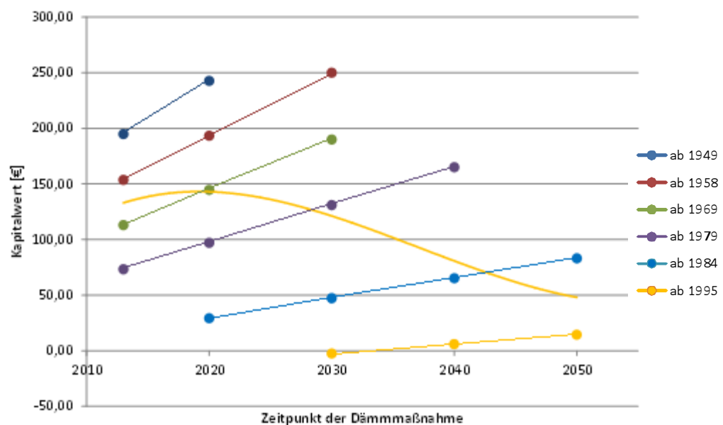
Abbildung 4.19: Trend des Kapitalwerts von Dämmmaßnahmen in Abhängigkeit von Zeitpunkt der Maßnahme und Baualter der Gebäude
