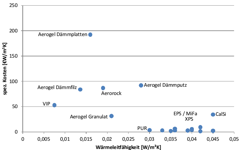
Abbildung 4.16: Spezifische Kosten verschiedener Dämmstoffe im Vergleich
