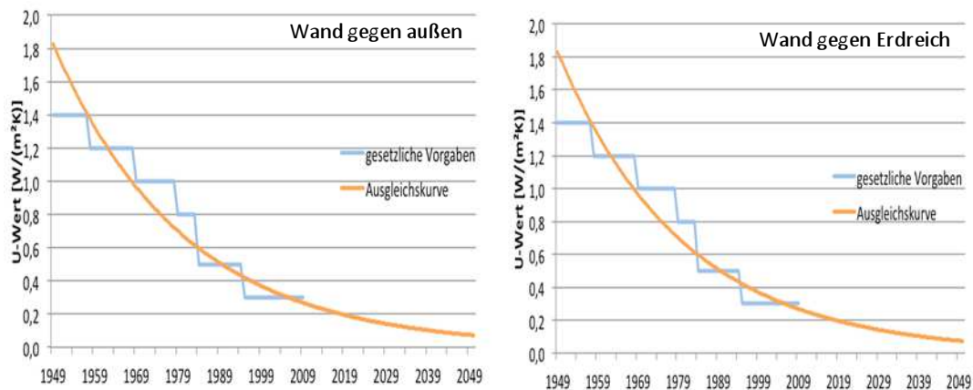
Abbildung 4.4: Extrapolation bisheriger U-Werte für die Bauteile Wand gegen außen (2050: U = 0,07 \text{ W/m}^2\text{K} ) und für die Bauteile Wand gegen Erdreich (2050: U = 0,07 \text{ W/m}^2\text{K} )
