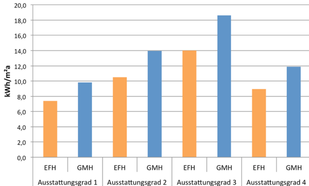
Abbildung 3.19: Darstellung Nutzwärmebedarf nach DIN 2067 Blatt 12 Tabelle 2
