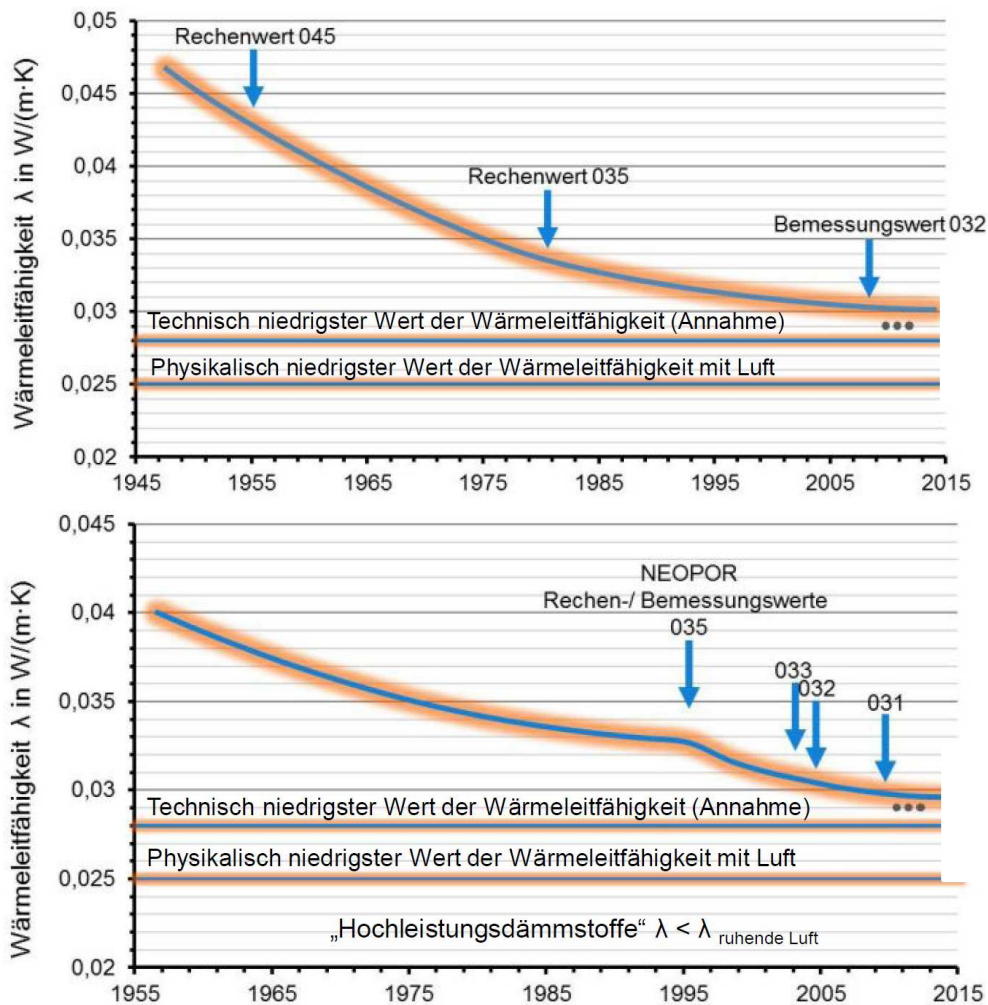
Abbildung 4.2: Entwicklung der Wärmeleitfähigkeiten von Mineralwolle und expandiertem Polystyrol in den vergangenen Dekaden (FTW, 2013)
