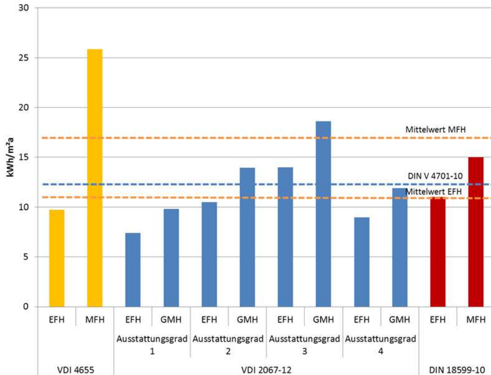
Abbildung 3.20: Darstellung Nutzwärmebedarf nach verschiedenen Regelwerken
