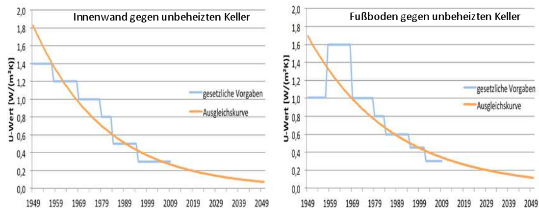
Abbildung 4.5: Extrapolation bisheriger U-Werte für die Bauteile Innenwand gegen unbeheizten Keller (2050: U = 0,07 \text{ W/m}^2\text{K} ) und für die Bauteile Fußboden gegen unbeheizten Keller (2050: U = 0,11 \text{ W/m}^2\text{K} )
