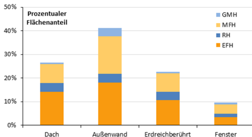
Abbildung 3.7: Prozentuale Verteilung der gesamten thermischen Hüllfläche auf die Bauteile Dach, Außenwand, erdbreichberührte Bauteile und Fenster im Jahr 2011, zusätzlich Differenzierung zwischen den Gebäudetypen
