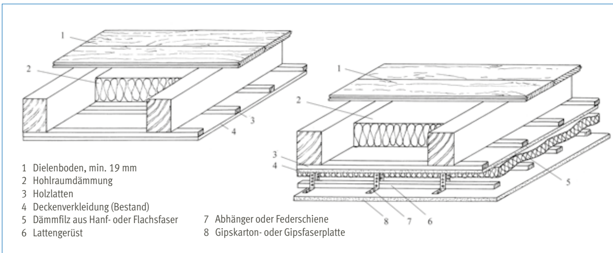
Rohboden: Holzbalkendecke mit Hohlraumdämmung und Gipskartondecke (links) Verbesserung von Schallschutz und Wärmeschutz auf der Deckenunterseite (rechts)
