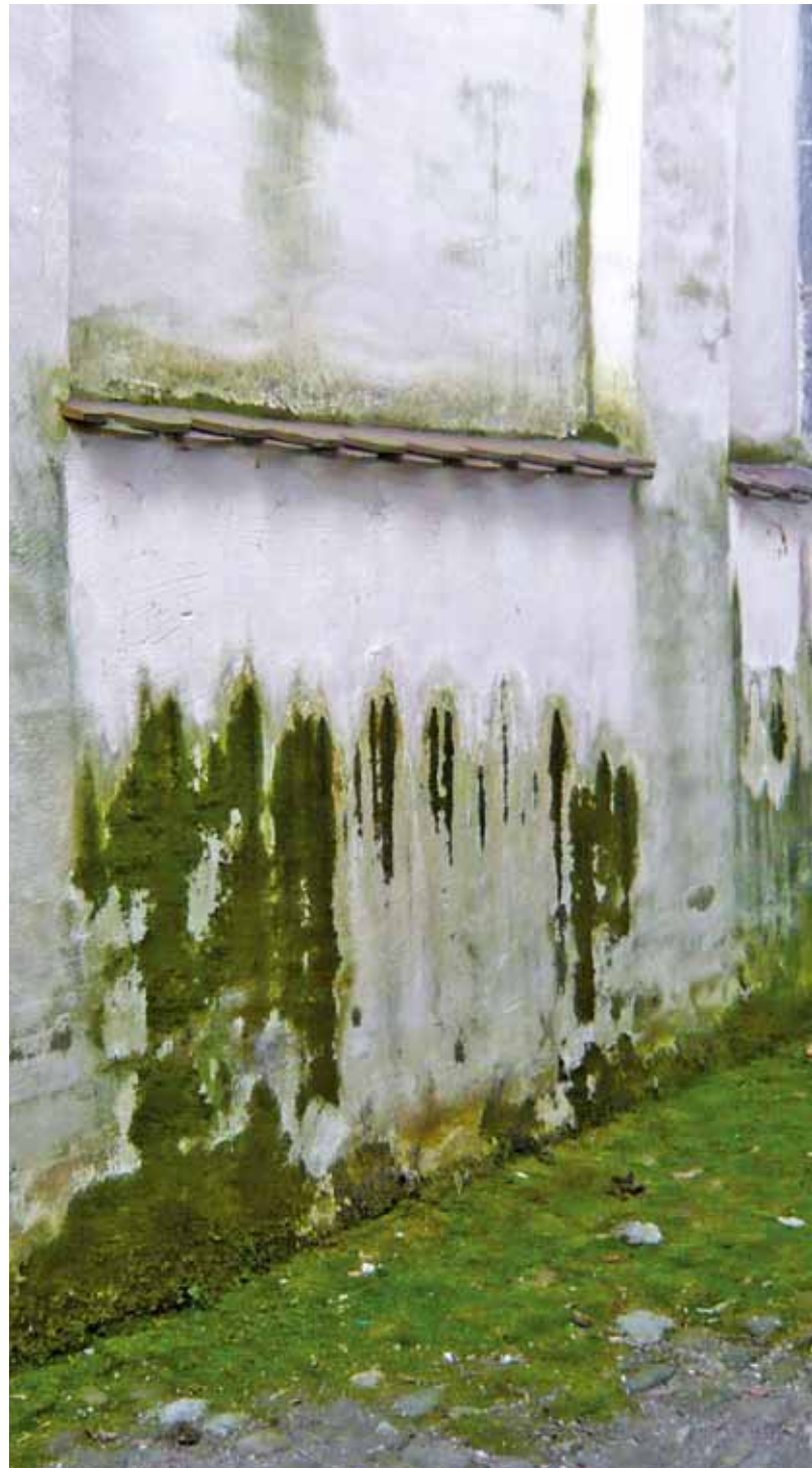
Aufsteigende Bodenfeuchte, Stauflüsse, Salzausblühungen, Algen- und Moosbewuchs – Faktoren aus unterschiedlichen Quellen wirken auf das Mauerwerk ein.
