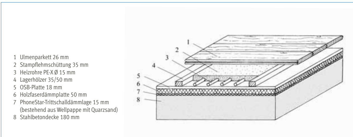
Betondecke mit Fußbodenheizung und Parkettboden auf Lagerhölzern
