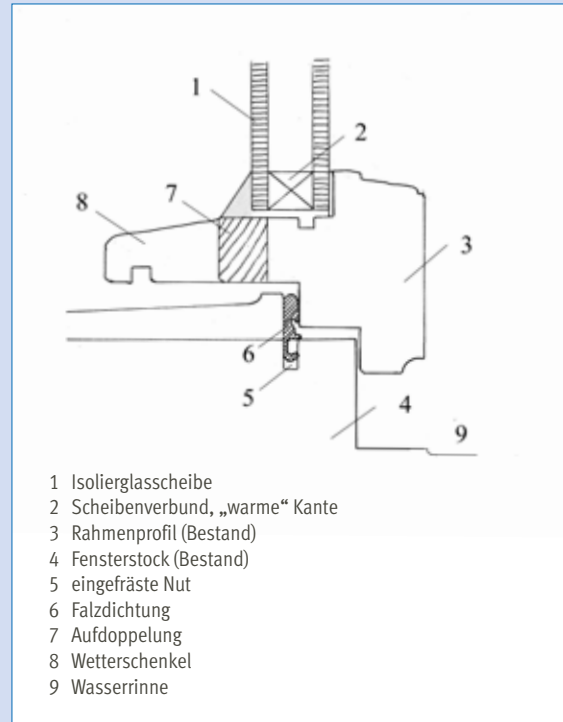
Thermische Verbesserung eines bestehenden Einfachglasfensters mit Isoliertglasscheibe
